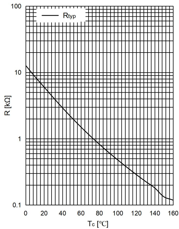
图 13 . 负温度系数热敏电阻 温度特性 Fig 13. NTC-Thermistor-temperature characteristic
