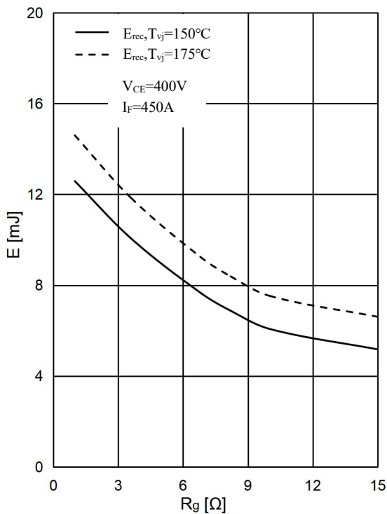
图 11 . 二极管 开关损耗-栅极电阻,逆变器 Fig 11. Diode Switching Loss E_{rec} vs. R_G ,Inverter
