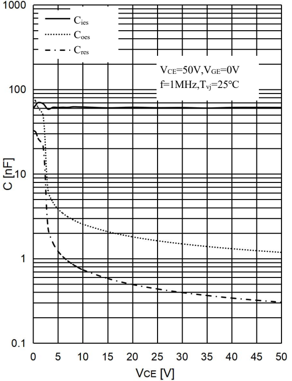
图 8 . IGBT 电容特性 Fig 8. IGBT Capacity Characteristic
