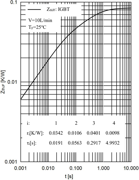
图 6 . IGBT 瞬态热阻抗 Fig 6. IGBT Transient thermal impedance
