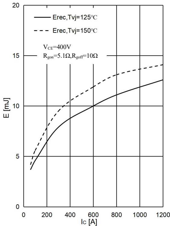
图 10 . 二极管 开关损耗-正向电流 Fig 10. Diode Switching Loss E_{rec} vs. I_F
