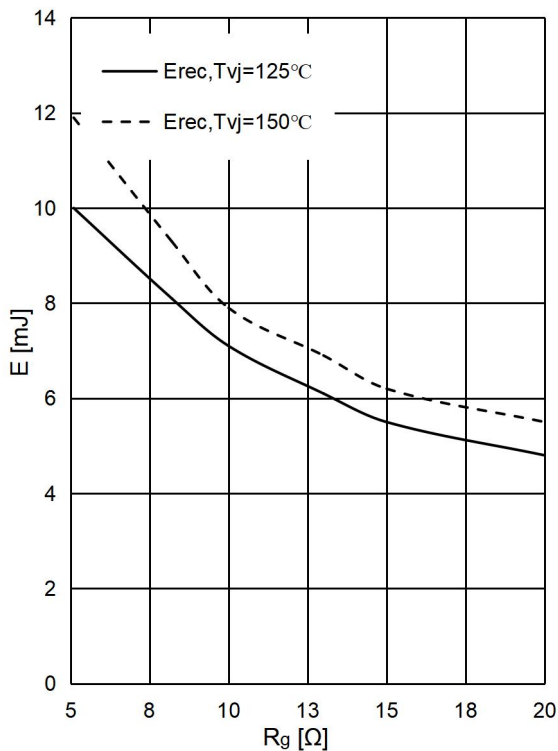
图 11 . 二极管 开关损耗-栅极电阻 Fig 11. Diode Switching Loss E_{rec} vs. R_G
