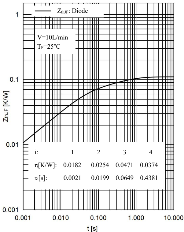
图 12 . 二极管 瞬态热阻抗 Fig 12. Diode Transient thermal impedance
