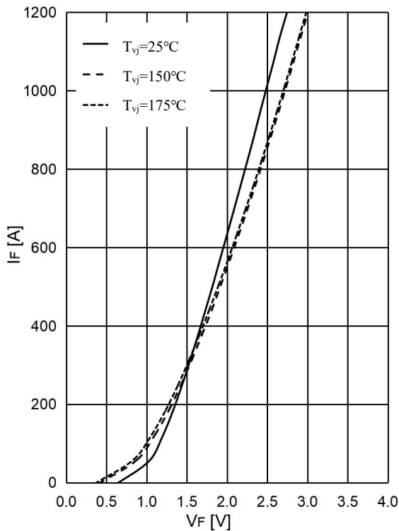
图 9 . 二极管 正向偏压特性 Fig 9. Diode Forward characteristic
