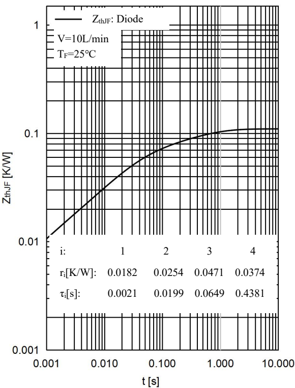
图 12 . 二极管 瞬态热阻抗,逆变器 Fig 12. Diode Transient thermal impedance,Inverter
