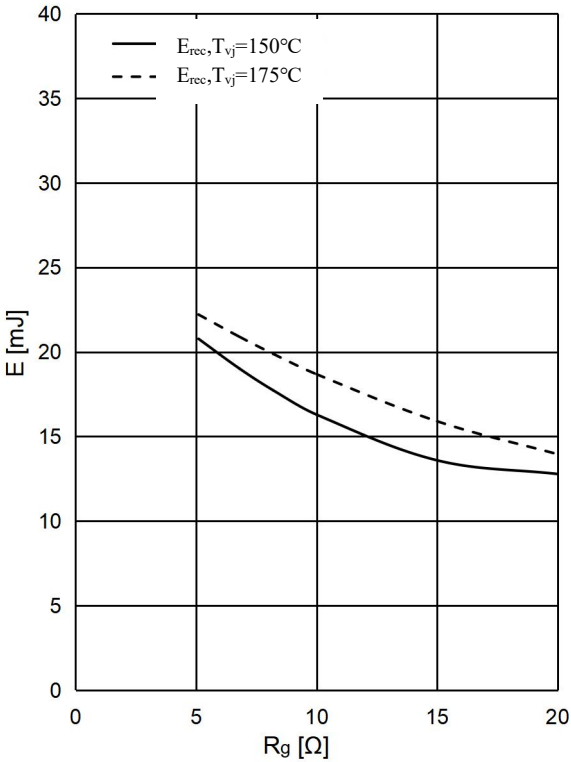
图 11 . 二极管 开关损耗-栅极电阻,逆变器 Fig 11. Diode Switching Loss E_{rec} vs. R_g ,InverterFig
