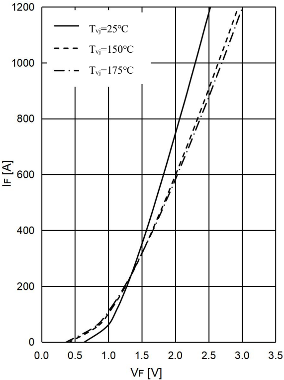
图 9 . 二极管 正向偏压特性,逆变器 Fig 9. Diode Forward characteristic,Inverter
