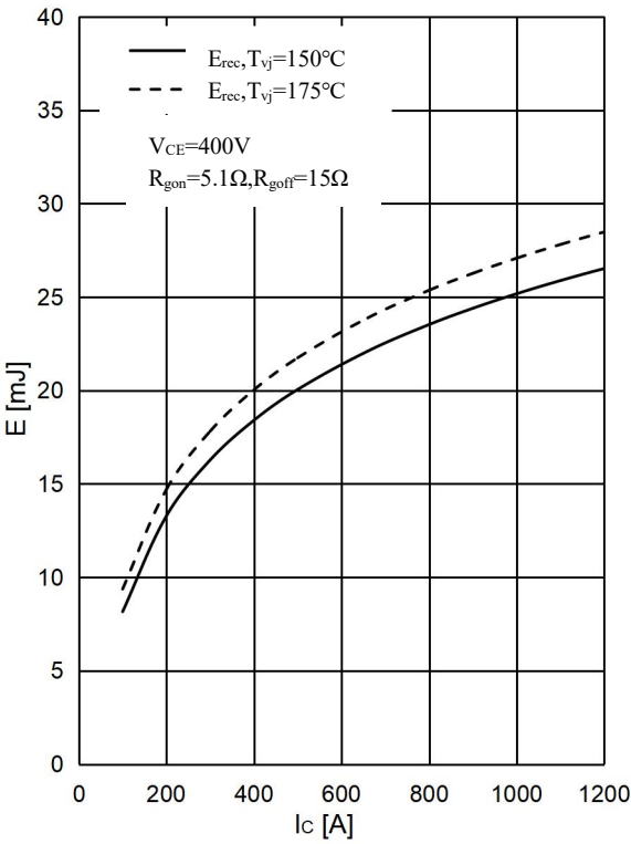
图 10 . 二极管 开关损耗-正向电流,逆变器 Fig 10. Diode Switching Loss E_{rec} vs. I_F ,Inverter
