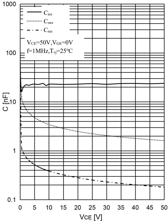
图 8 . IGBT 电容特性,逆变器 Fig 8. IGBT Capacity Characteristic, Inverter
