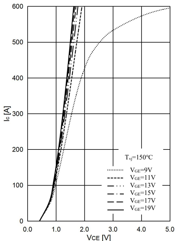
图 2 . IGBT 输出特性,逆变器
