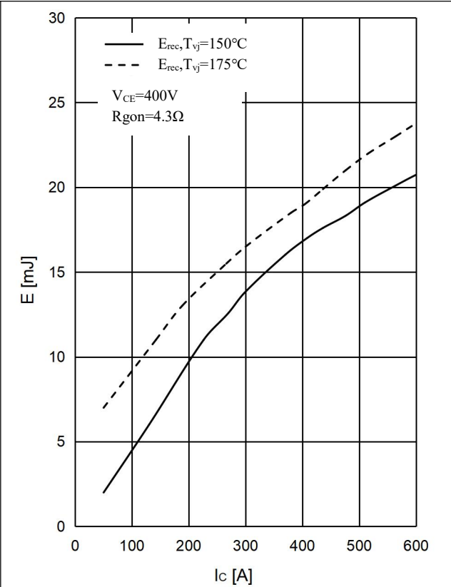
图 9 . 二极管 开关损耗-正向电流,逆变器 Fig 9. Diode Switching Loss Erec vs. IF,Inverter
