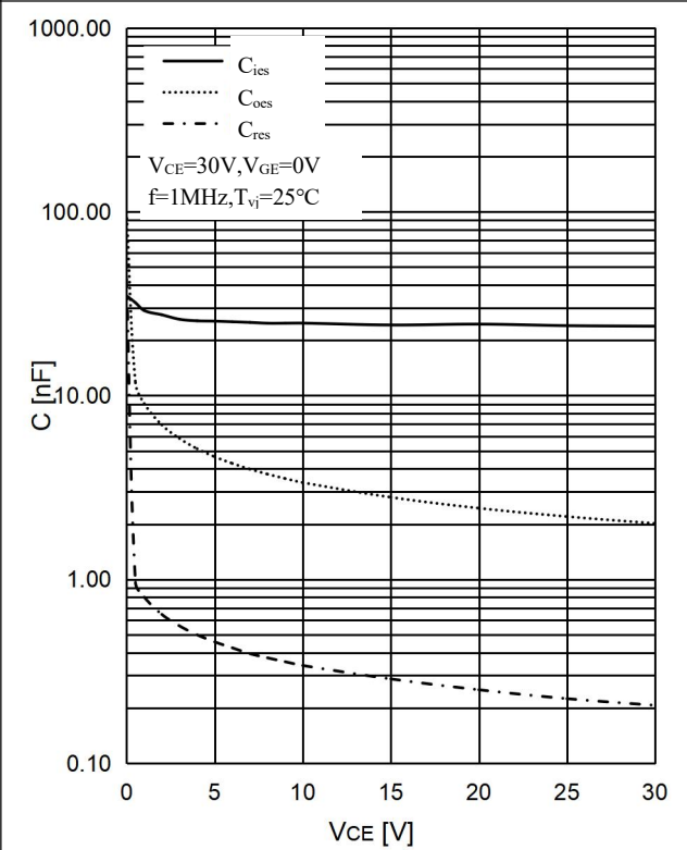
图 8 . IGBT 电容特性,逆变器 Fig 8. IGBT Capacity Characteristic, Inverter
