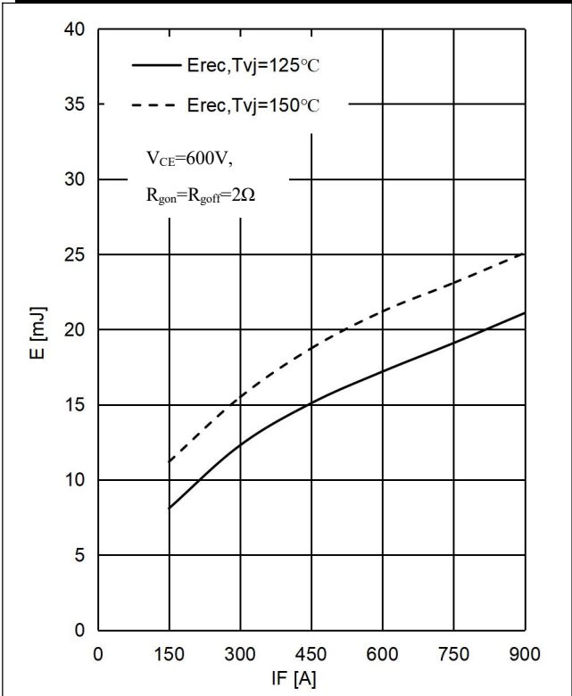
图 9 . 二极管 开关损耗-正向电流 Fig 9. Diode Switching Loss E_{rec} vs. I_F
