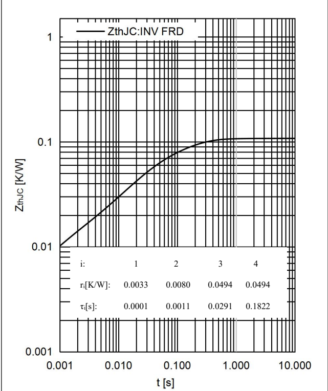
图 11 . 二极管 瞬态热阻抗 Fig 11. Diode Transient thermal impedance
