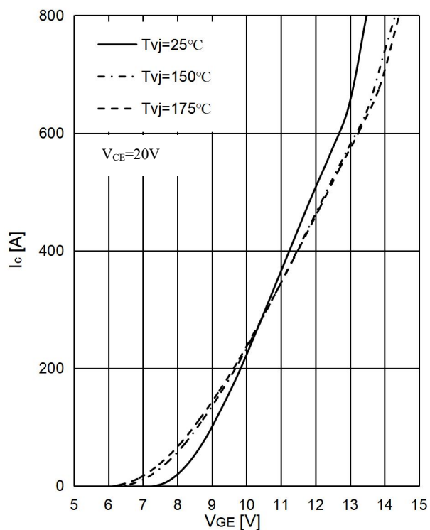
图 3 . IGBT 转移特性
