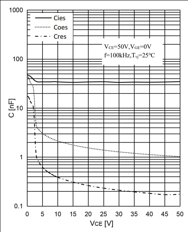
图 8 . IGBT 电容特性 Fig 8. IGBT Capacity Characteristic
