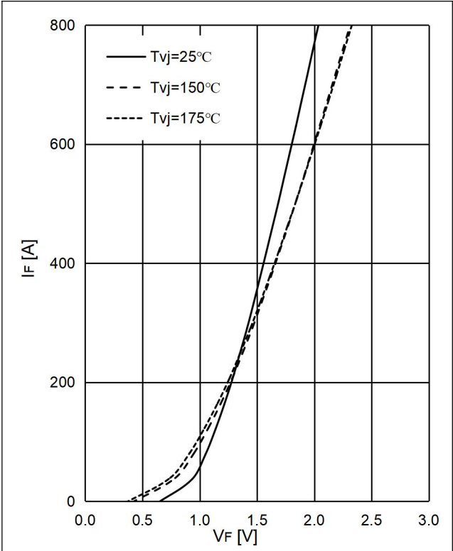
图 9 . 二极管 正向偏压特性 Fig 9. Diode Forward characteristic
