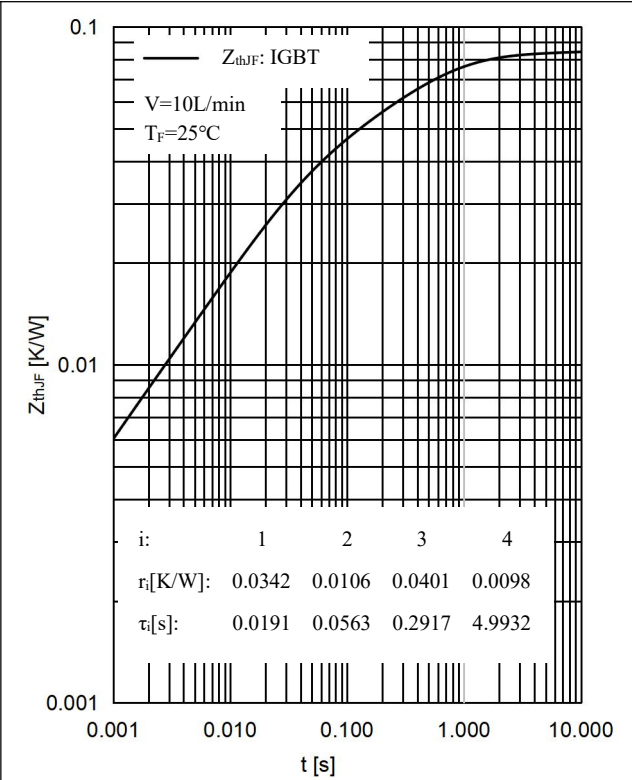
图 6 . IGBT 瞬态热阻抗 Fig 6. IGBT Transient thermal impedance
