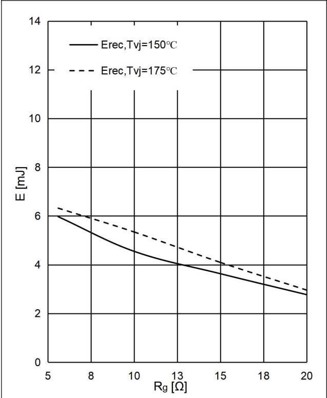
图 11 . 二极管 开关损耗-栅极电阻 Fig 11. Diode Switching Loss E_{rec} vs. R_g
