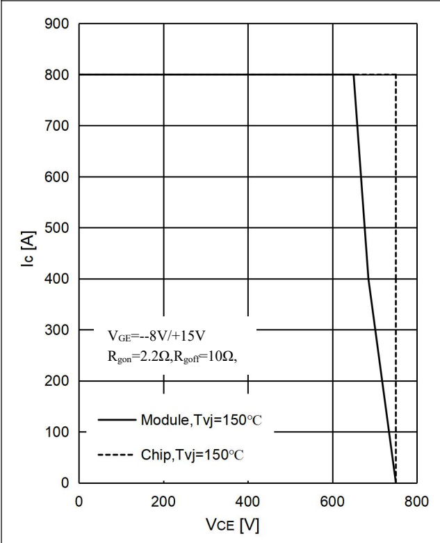
图 7 . IGBT 反偏安全工作区 Fig 7. IGBT RBSOA
