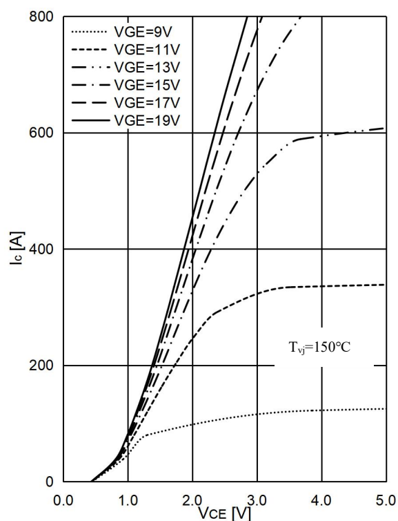
图 2 . IGBT 输出特性
