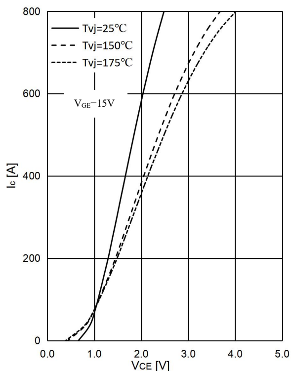
图 1 . IGBT 输出特性
