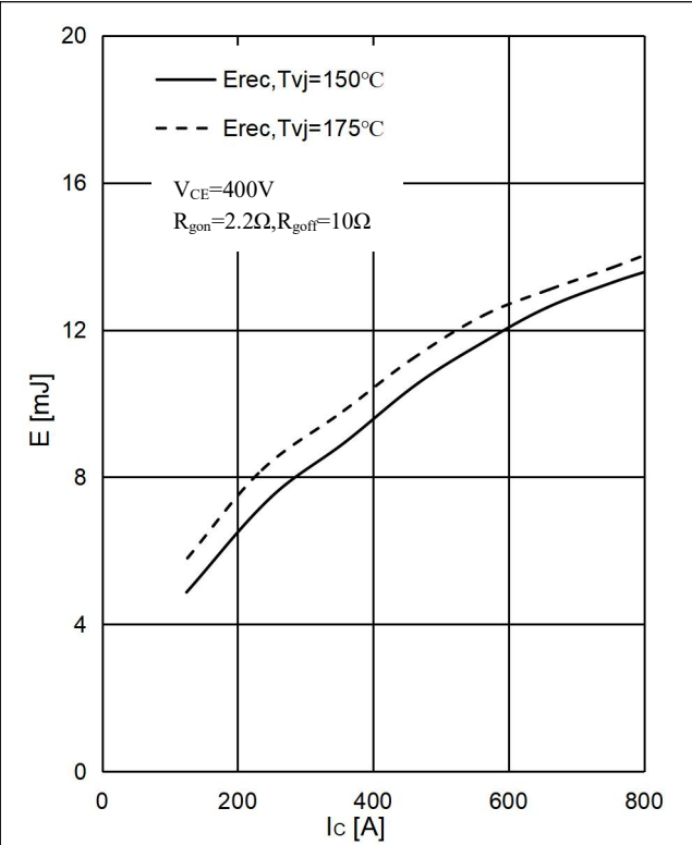
图 10 . 二极管 开关损耗-正向电流 Fig 10. Diode Switching Loss E_{rec} vs. I_F
