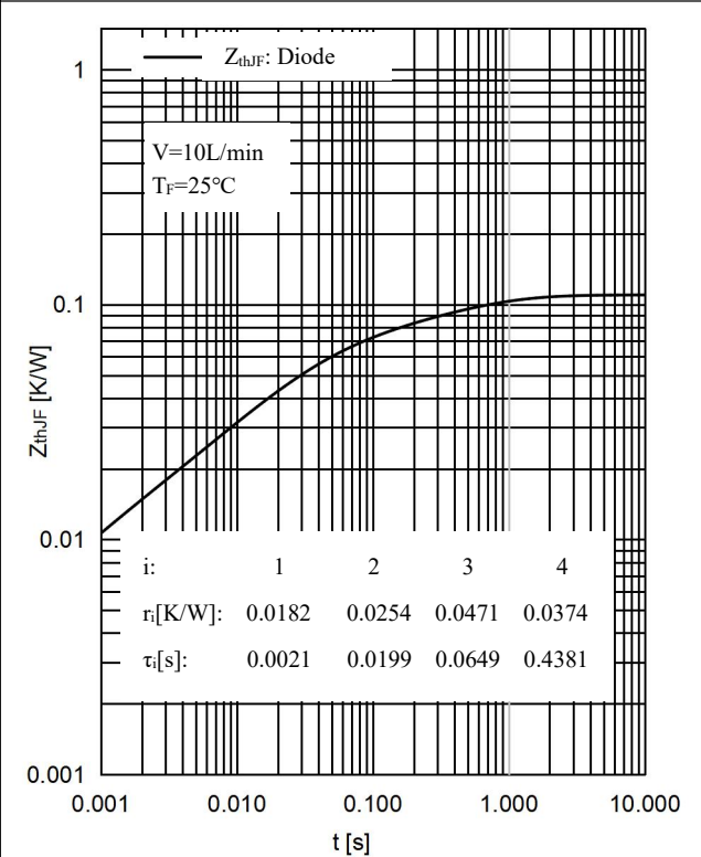
图 12 . 二极管 瞬态热阻抗 Fig 12. Diode Transient thermal impedance
