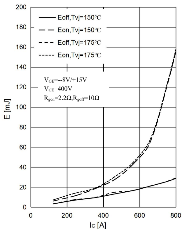
图 4 . IGBT 开关损耗-集电极电流
