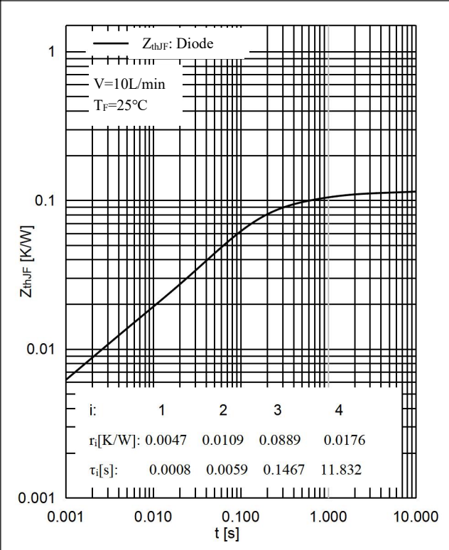
图 12 . 二极管 瞬态热阻抗,逆变器 Fig 12. Diode Transient thermal impedance,Inverter
