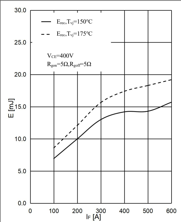
图 10 . 二极管 开关损耗-正向电流,逆变器 Fig 10. Diode Switching Loss E_{rec} vs. I_F ,Inverter
