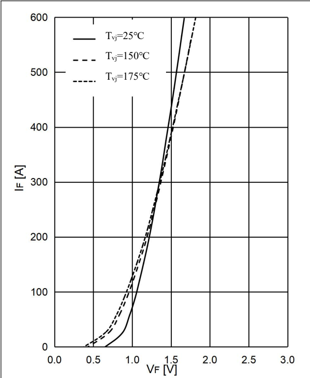
图 9 . 二极管 正向偏压特性,逆变器 Fig 9. Diode Forward characteristic,Inverter
