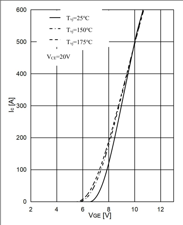
图 3 . IGBT 转移特性,逆变器 Fig 3. IGBT Transfer Characteristic,Inverter
