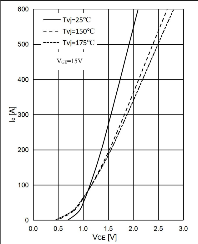
图 1 . IGBT 输出特性,逆变器 Fig 1. IGBT Output Characteristic,Inverter
