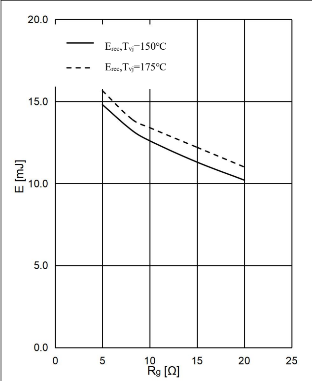
图 11 . 二极管 开关损耗-栅极电阻,逆变器 Fig 11. Diode Switching Loss E_{rec} vs. R_g ,InverterFig
