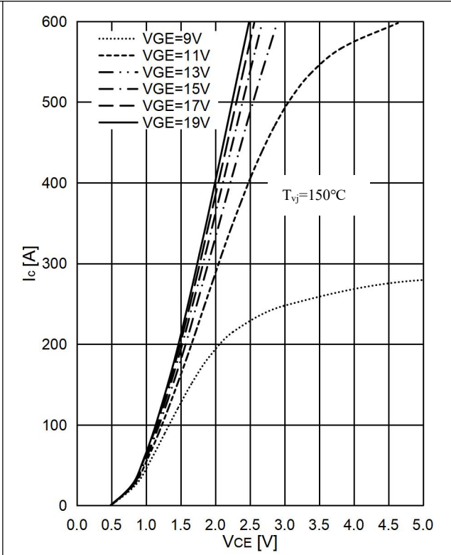
图 2 . IGBT 输出特性,逆变器 Fig 2. IGBT Output Characteristic,Inverter
