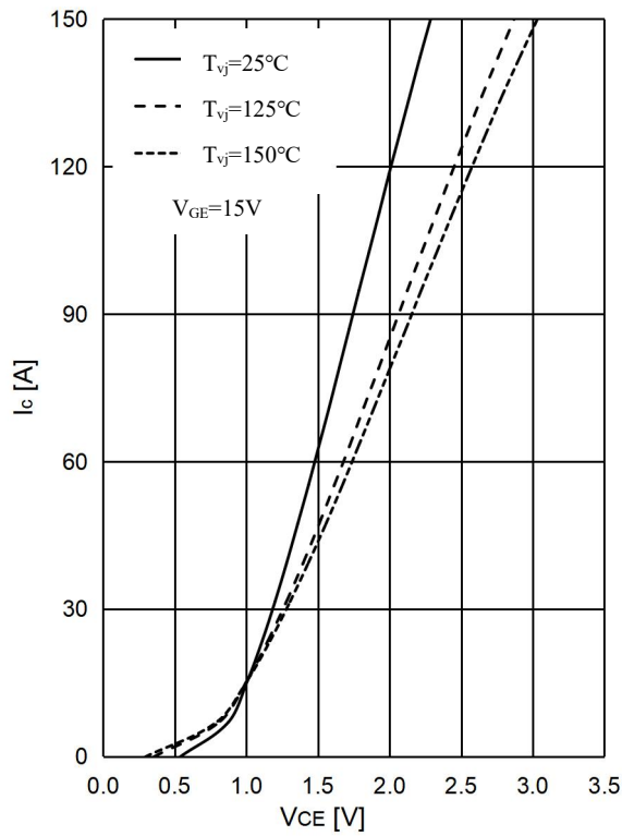
图 1 . IGBT 输出特性,逆变器
