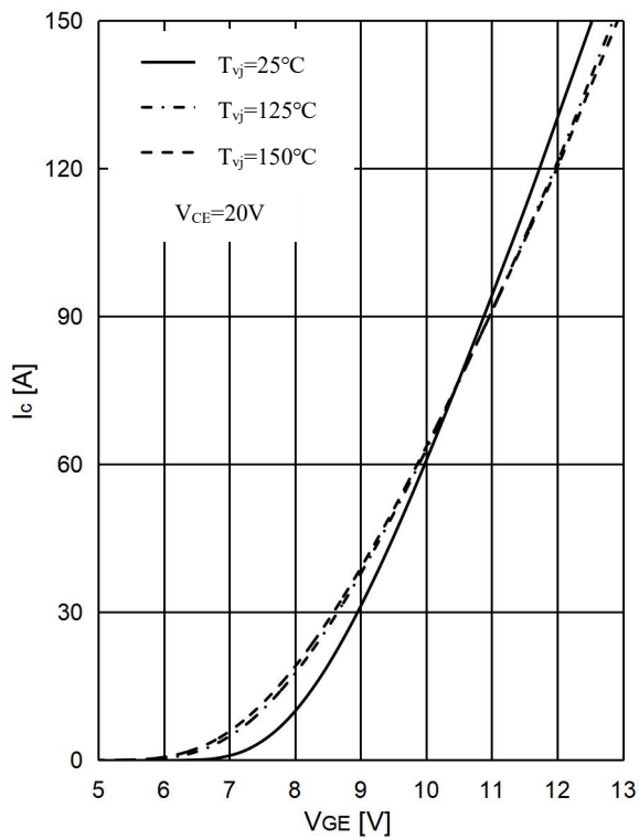
图 3 . IGBT 转移特性,逆变器
