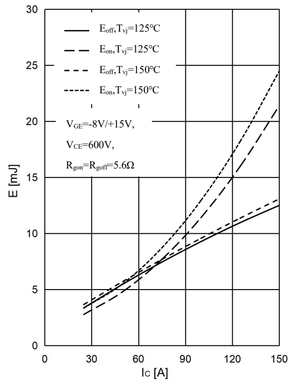
图 4 . IGBT 开关损耗-集电极电流,逆变器
