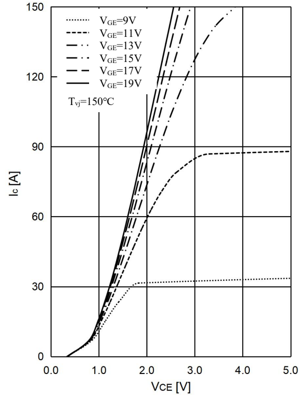
图 2 . IGBT 输出特性,逆变器
