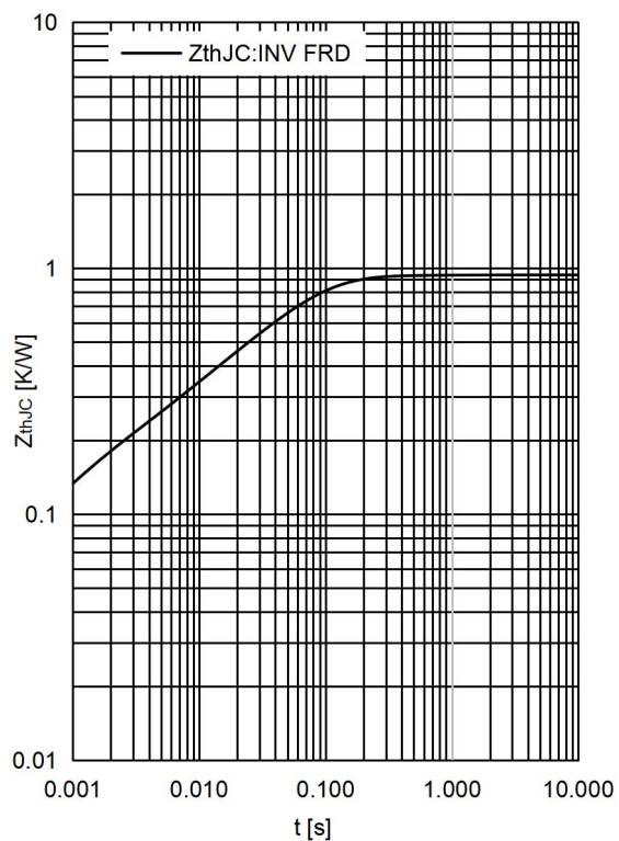
图 11 . 二极管 瞬态热阻抗,逆变器
