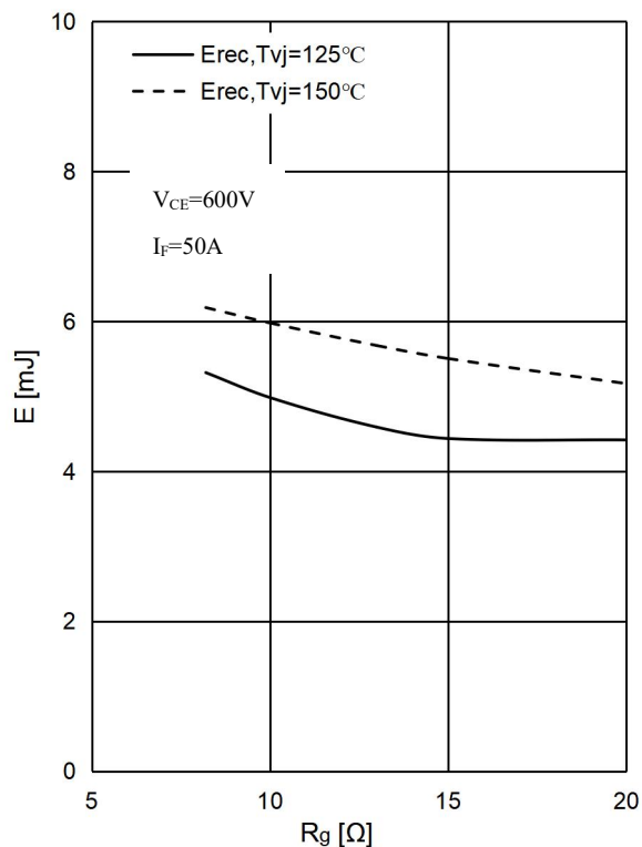
图 10 . 二极管 开关损耗-栅极电阻,逆变器
