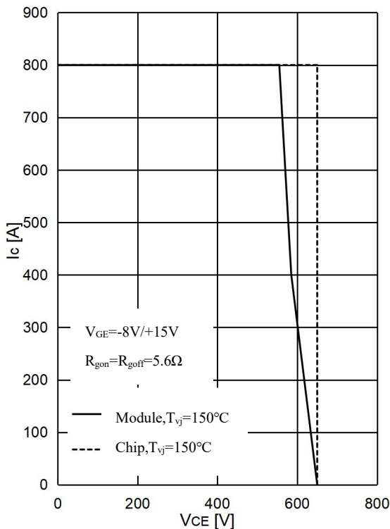
图 7 . IGBT 反偏安全工作区,T1&T2&T3&T4 Fig 7. IGBT RBSOA
