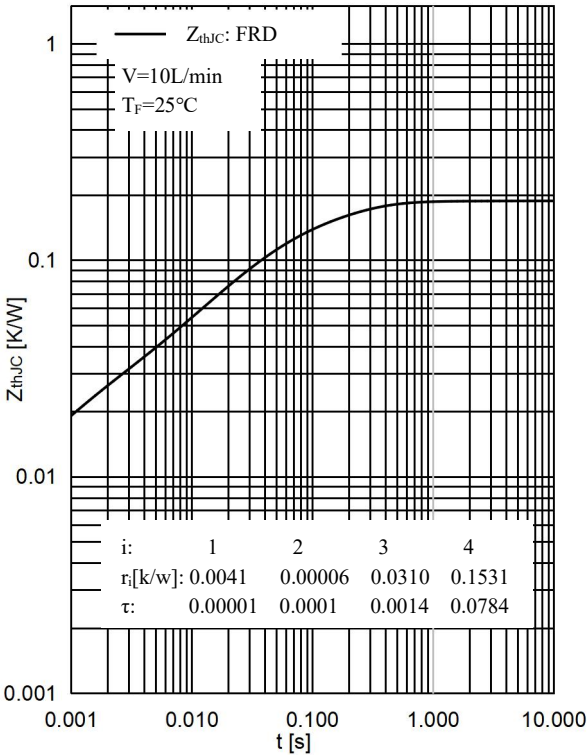
图 12 . 二极管 D1&D2&D3&D4 瞬态热阻抗 Fig 12. Diode D1&D2&D3&D4 Transient thermal impedance
