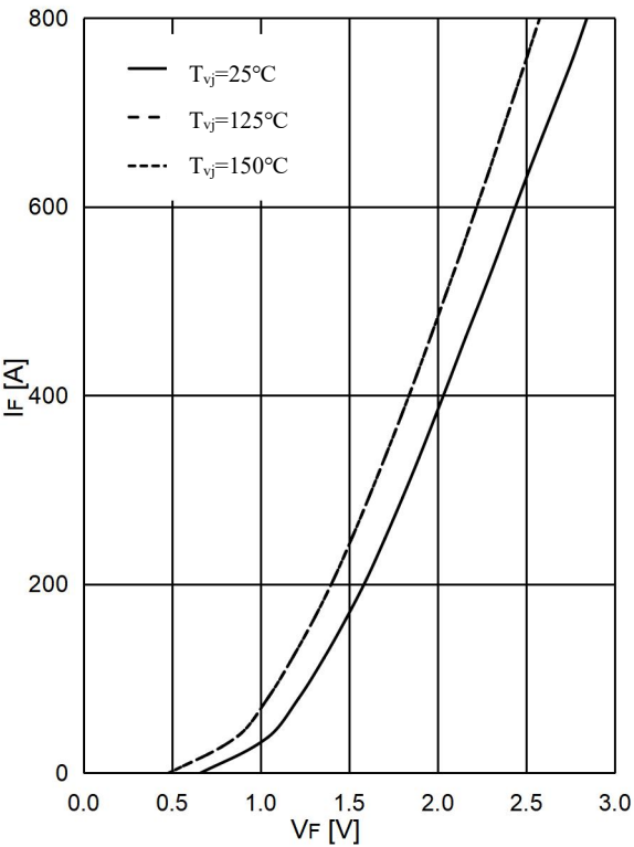
图 9 . 二极管 D1&D2&D3&D4 正向偏压特性 Fig 9 . Diode D1&D2&D3&D4 Forward characteristic
