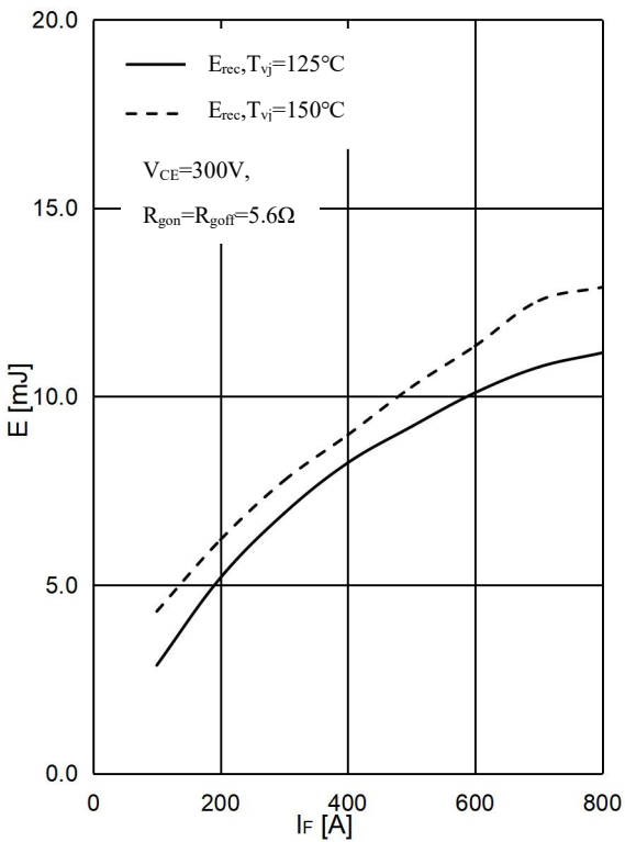
图 10 . 二极管 D1&D2&D3&D4 开关损耗-正向电流 Fig 10. Diode D1&D2&D3&D4 Switching Loss E_{rec} vs. I_F
