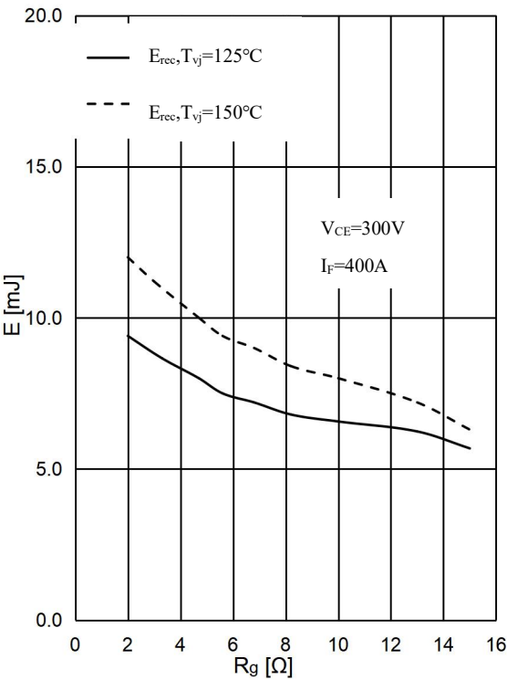
图 11 . 二极管 D1&D2&D3&D4 开关损耗-栅极电阻 Fig 11. Diode D1&D2&D3&D4 Switching Loss E_{rec} vs. R_G
