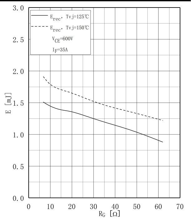
图 10 . 二极管 开关损耗-栅极电阻,逆变器 Fig 10. Diode Switching Loss E_{rec} vs. R_G ,Inverter
