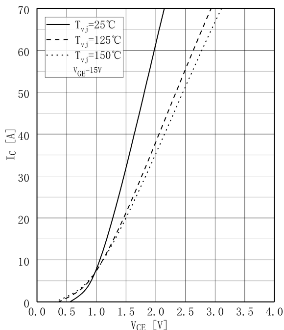
图 1 . IGBT 输出特性,逆变器 Fig 1. IGBT Output Characteristic, Inverter
