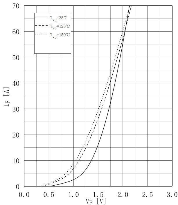
图 8 . 二极管 正向偏压特性,逆变器 Fig 8. Diode Forward characteristic, Inverter
