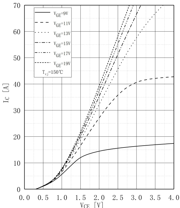
图 2 . IGBT 输出特性,逆变器 Fig 2. IGBT Output Characteristic, Inverter
