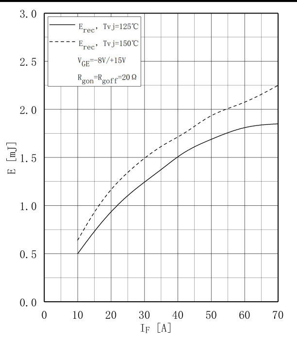
图 9 . 二极管 开关损耗-正向电流,逆变器 Fig 9. Diode Switching Loss E_{rec} vs. I_F ,Inverter
