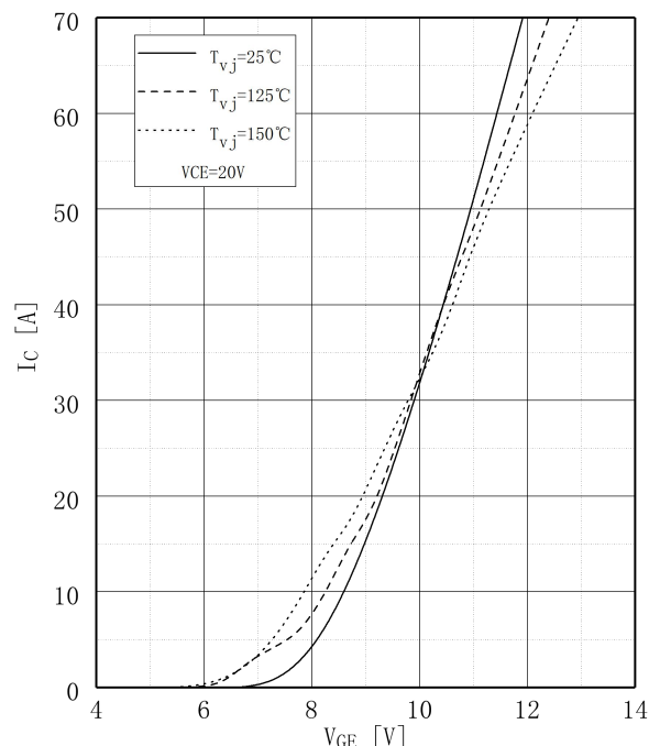
图 3 . IGBT 转移特性,逆变器 Fig 3. IGBT Transfer Characteristic, Inverter
