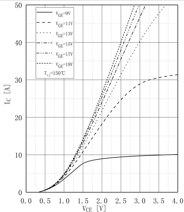
图 2 . IGBT 输出特性,逆变器
