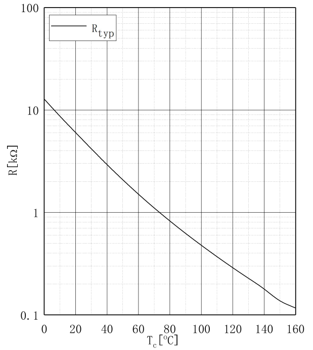
图 12 . 负温度系数热敏电阻 温度特性 Fig 12. NTC-Thermistor-temperature characteristic
