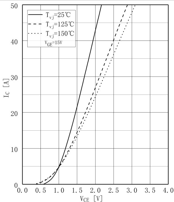
图 1 . IGBT 输出特性,逆变器
