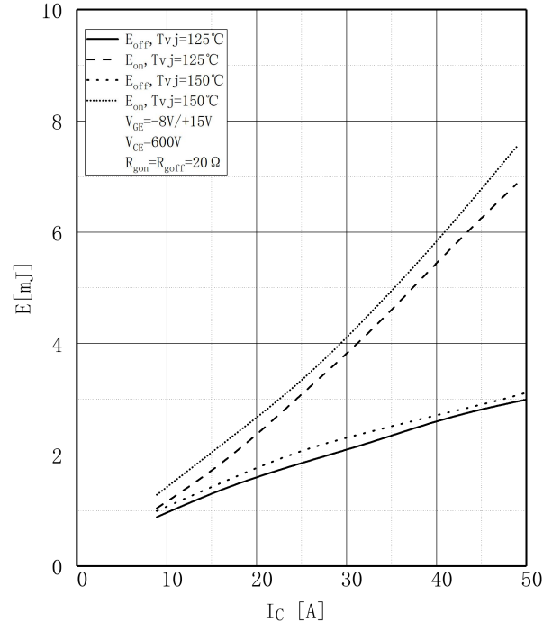
图 4 . IGBT 开关损耗-集电极电流,逆变器
