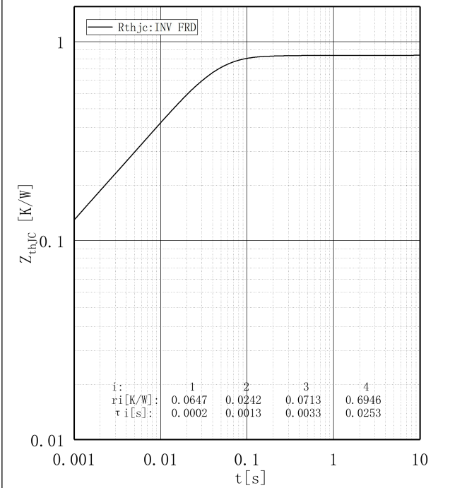
图 11 . 二极管 瞬态热阻抗,逆变器 Fig 11. Diode Transient thermal impedance,Inverter
