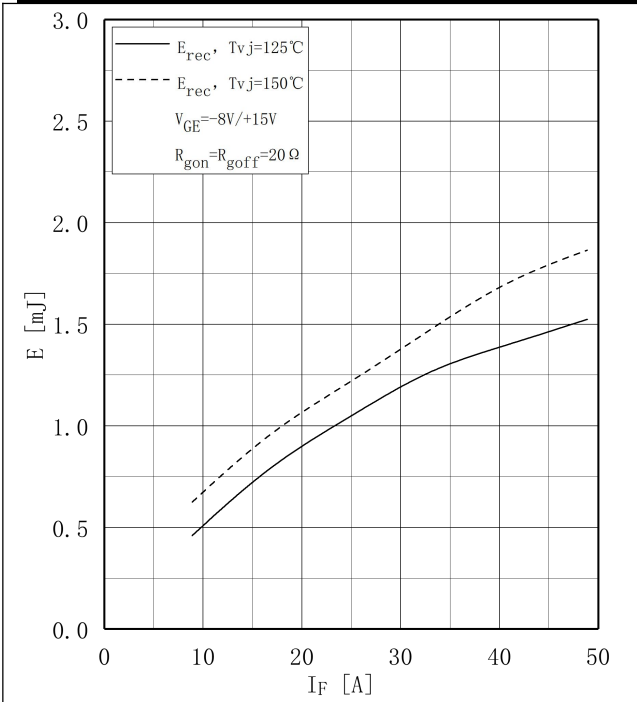
图 9 . 二极管 开关损耗-正向电流,逆变器 Fig 9. Diode Switching Loss E_{rec} vs. I_F ,Inverter
