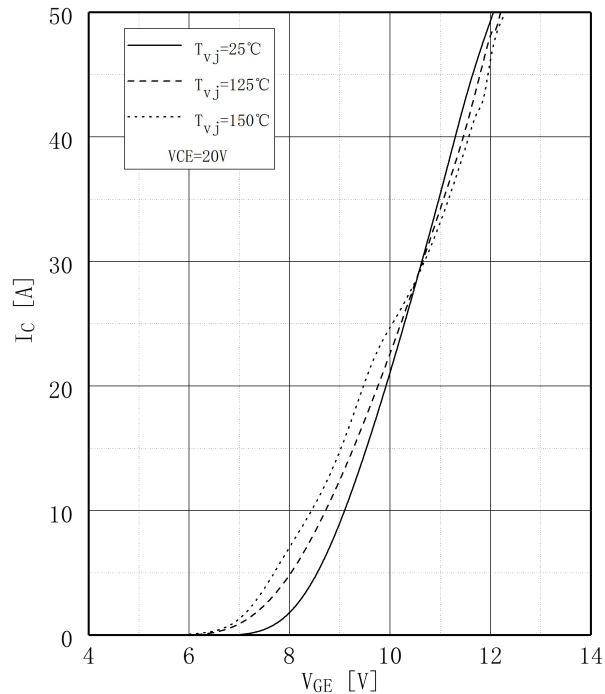
图 3 . IGBT 转移特性,逆变器
