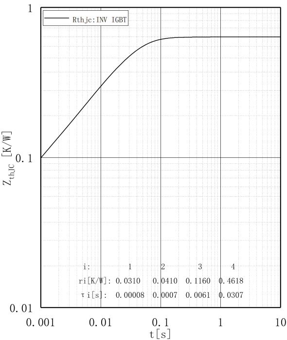
图 6 . IGBT 瞬态热阻抗,逆变器 Fig 6. IGBT Transient thermal impedance,Inverter
