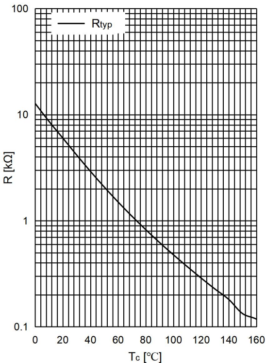
图 12 . 负温度系数热敏电阻 温度特性 Fig 12. NTC-Thermistor-temperature characteristic
