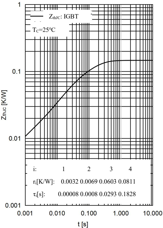
图 6 . IGBT 瞬态热阻抗,逆变器 Fig 6. IGBT Transient thermal impedance, Inverter
