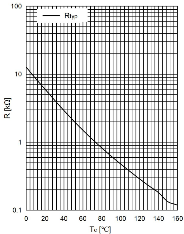
图 12. 负温度系数热敏电阻 温度特性
