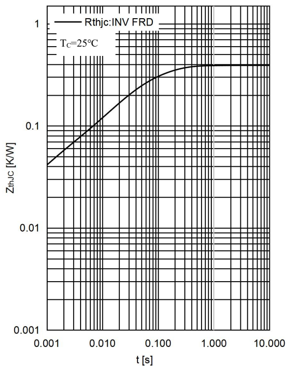
图 11. 二极管 瞬态热阻抗,逆变器
