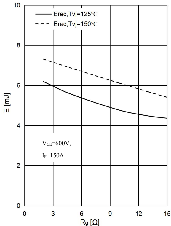
图 10. 二极管 开关损耗-栅极电阻,逆变器
