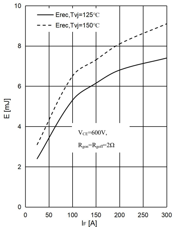
图 9. 二极管 开关损耗-正向电流,逆变器
