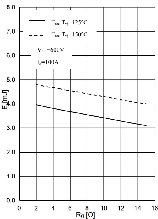
图 10 . 二极管 开关损耗-栅极电阻,逆变器 Fig 10. Diode Switching Loss E_{rec} vs. R_G , Inverter
