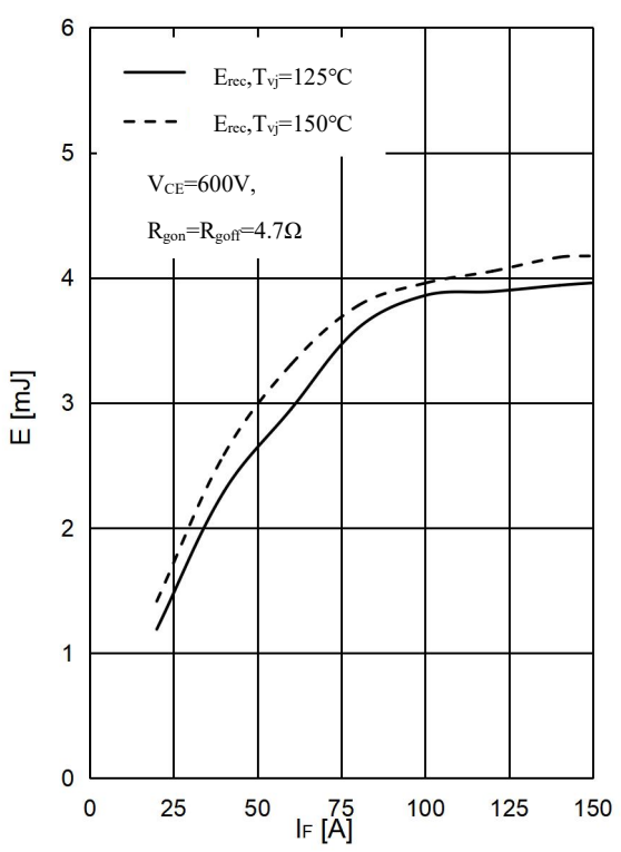
图 8 . 二极管 开关损耗-正向电流,逆变器 Fig 8. Diode Switching Loss E_{rec} vs. I_F , Inverter
